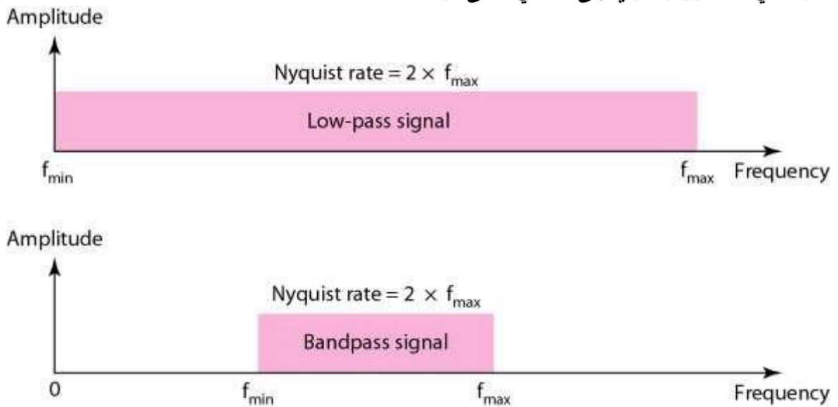
الشكل-13: معدل العينة لإشارة تمرير منخفض وإشارة تمرير حزمة.
